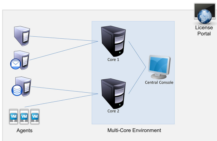
図 3. AppAssure 5 の複数コアの展開アーキテクチャ
