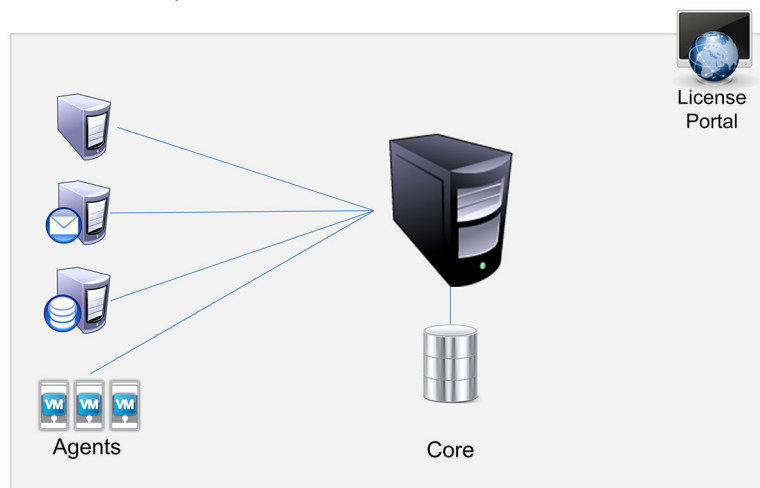
図 2. AppAssure 5 の基本的な展開アーキテクチャ
