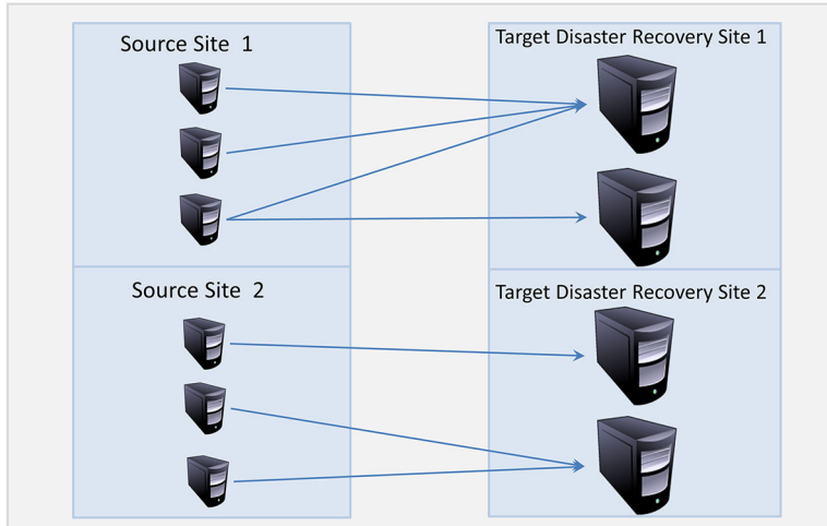
図 9. マルチポイント複製アーキテクチャの図
