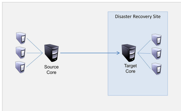
図 5. 基本的な複製アーキテクチャ
