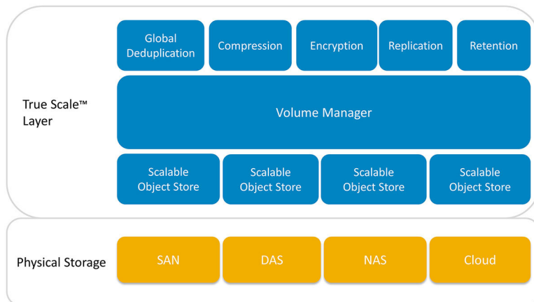
図 1. AppAssure True Scale アーキテクチャ
